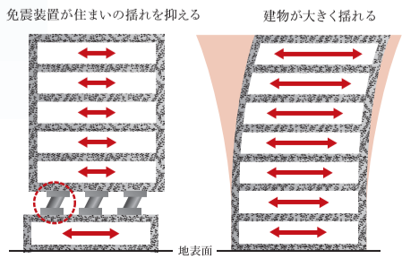
本物件採用の免震構造
